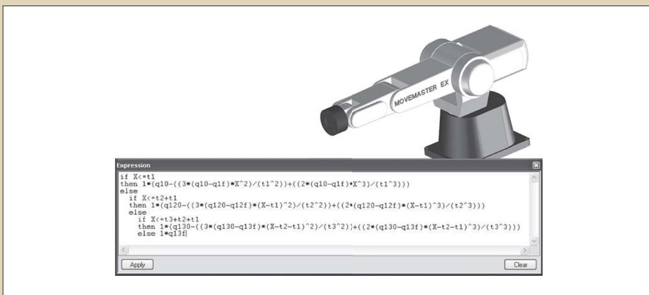
Rys. 2. Zapis równań ruchu robota Movemaster.
